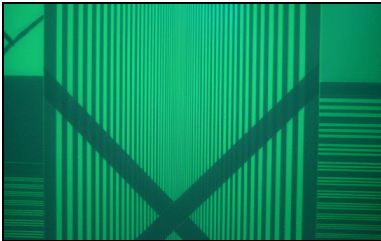
Рис. 4. Съемка X-Ray тест Siemens на CMOS камеру на микрофокусном рентгеновском аппарате. Выделен фрагмент теста H*V = 56 * 35 mm (пиксель \sim 56\mu\text{m} ).
