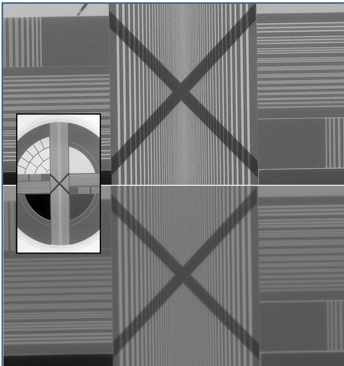
Рис. 1. X-Ray тест Siemens, соответствует легким среднему пациента, режим 60kV/20mAs . Выделен фрагмент теста H*V = 73*29mm (пиксель \approx 85\mu m ), фокус 0.5*0.5mm . Внизу исходное изображение, вверху – после многоступенчатой обработки, видимое разрешение до 0.25mm, слева полное изображение теста Siemens.
